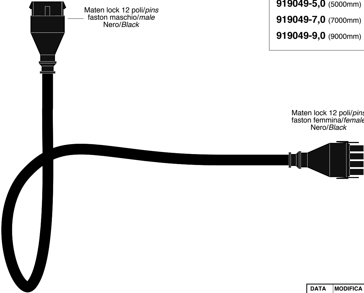
Maten lock 12 poli/pins faston maschio/male Nero/Black
