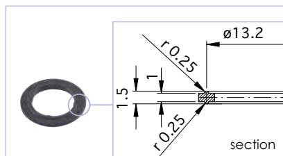
cod. 250076 - Shore A: 75
